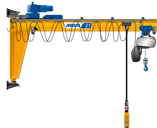
Fig.: VW con accesorios (motor eléctrico de giro y botonera colgante desplazable)
